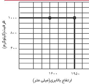
منحنی ظرفیت
